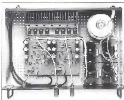
Compleet gemonteerde A-18 versterker
